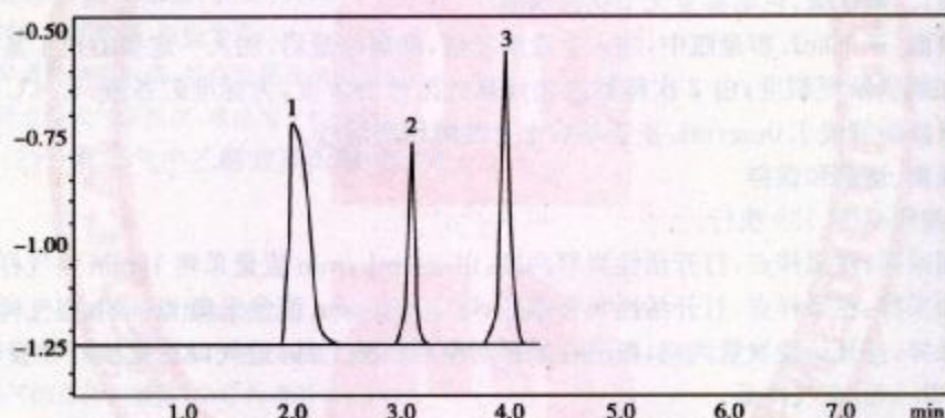
图 1 色谱分离图
